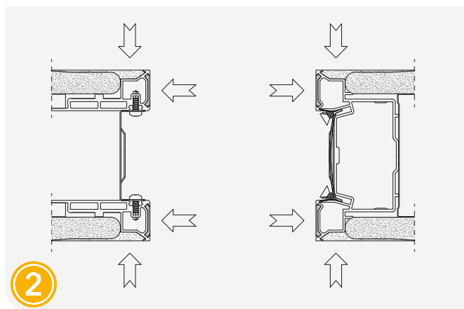
Nanesi gips na profil obeh pokončnikov
