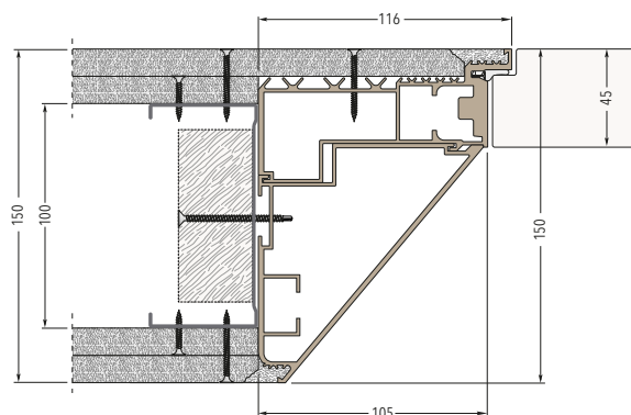
Z dvema mavčnima ploščama: Debelina končne stene 150 mm
