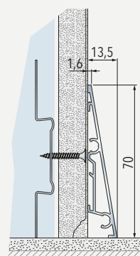
PODBOJ MAVČNA PLOŠČA
