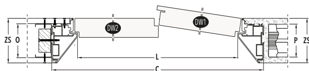
VRATA NA POTISK
