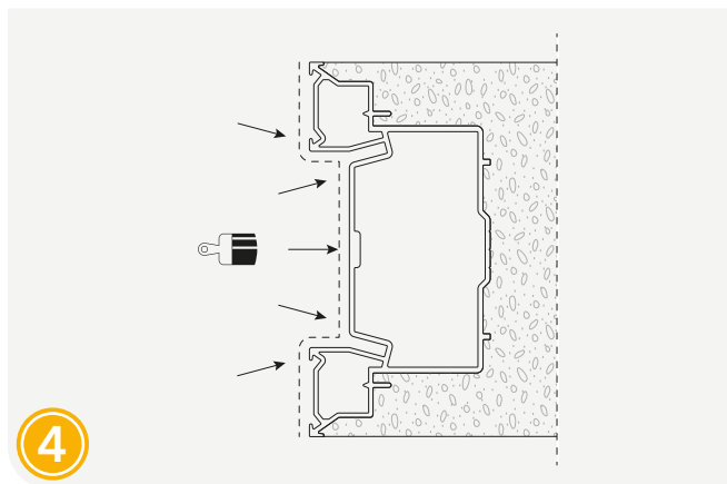
Odstrani PVC zaščito na pokončniku in pobarvaj.
