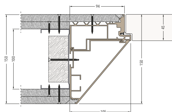
Z dvema mavčnima ploščama: Debelina končne stene 150 mm
