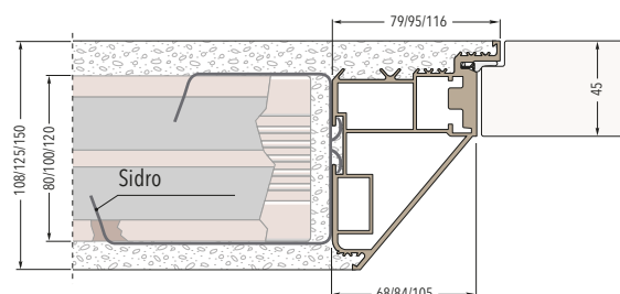
VRATA NA VLEKO
