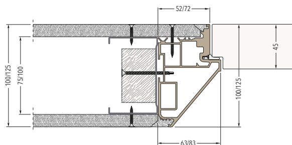
Z dvema mavčnima ploščama: Debelina končne stene 125 mm
