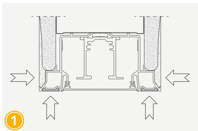
Nanesi gips na profil prečnika
