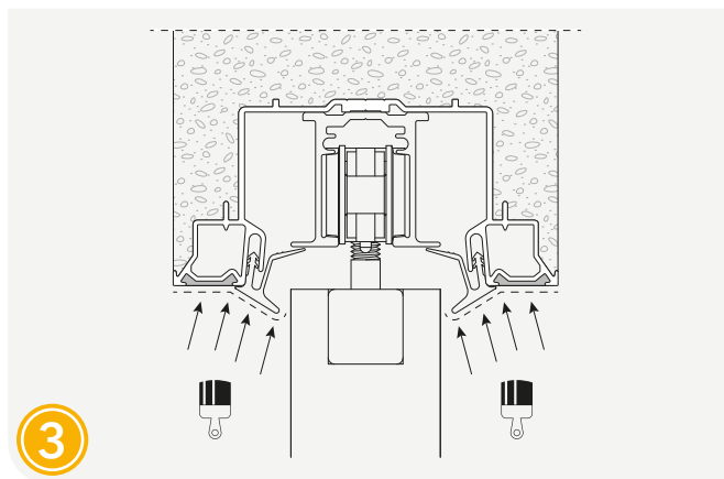
Odstrani zaščito in vstavi tesnila. Pobarvaj tesnilo na prečniku.
