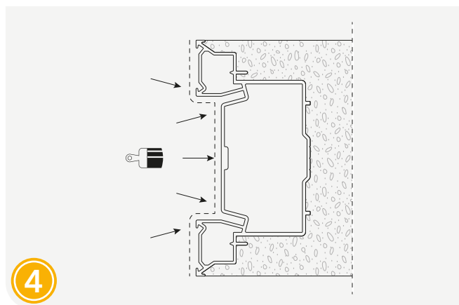
Uklonite PVC zaštitu na vertikalnom profilu i obojajte.
