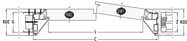
VRATA NA GURANJE
