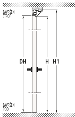
VRATA NA GURANJE
