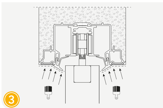
Uklonite zaštitu i umetnite brtvu. Obojaj brtvu na traverzi.
