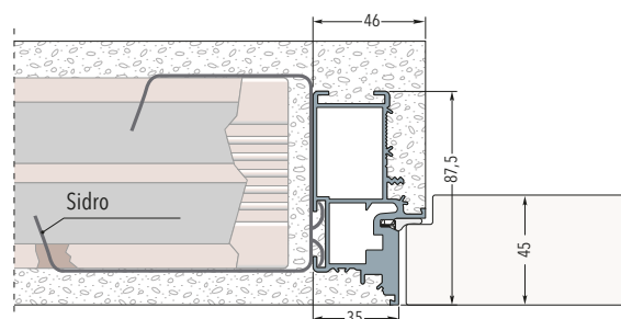
VRATA NA POVLAČENJE
