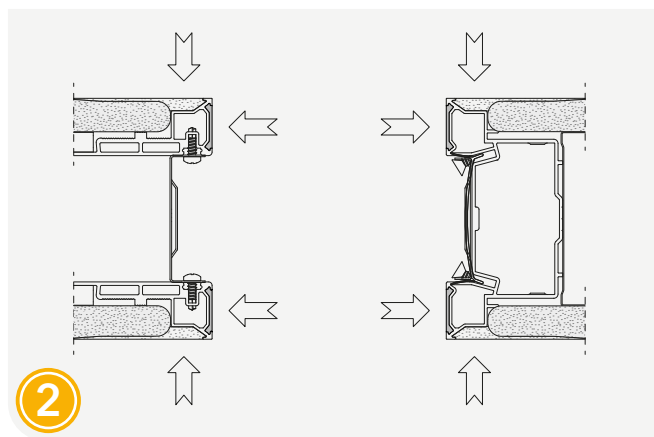
Podletaj oba vertikalna profila.
