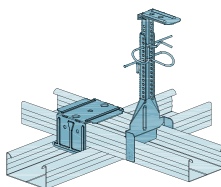
Rigips Nonius-sistem z Rigips križno vezjo
