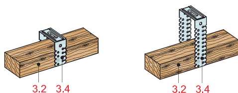
Rigips direktno obešalo
