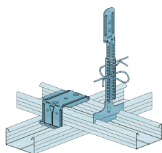
Rigips Nonius-sistem z Rigips križno vezjo
